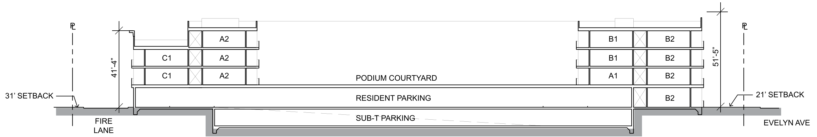
SITE SECTION A-A
