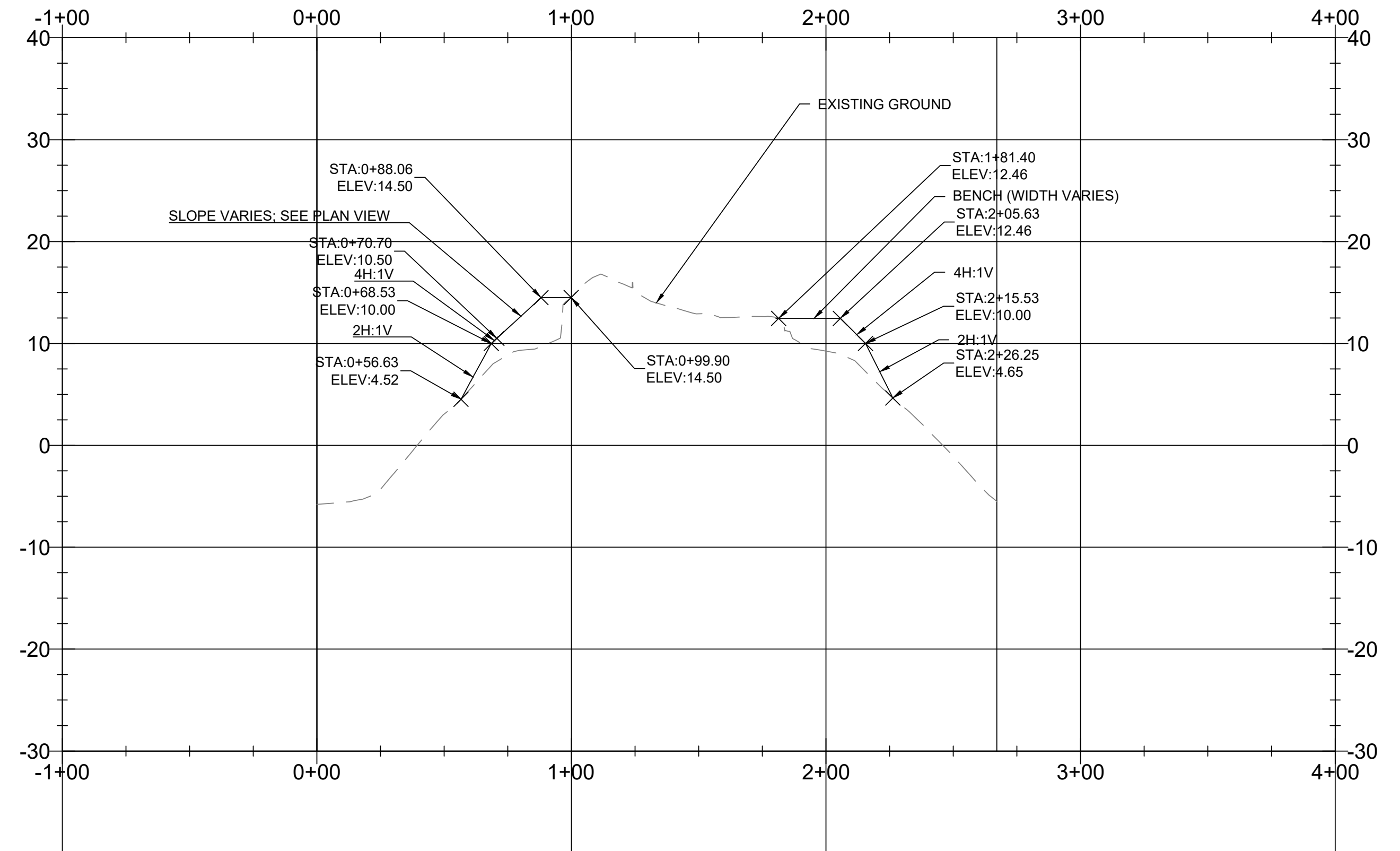
A SECTION A-A SCALE: 1" = 40' (HRZ), 1"=10' (VRT)
