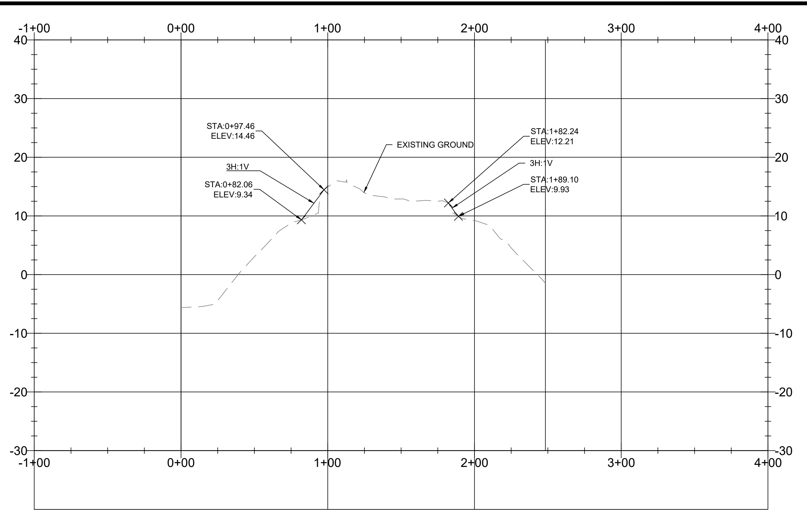
A SECTION A-A SCALE: 1" = 40' (HRZ), 1"=10' (VRT)
